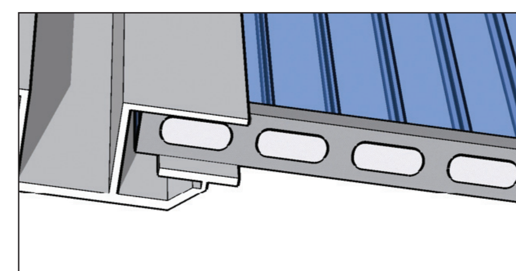
AD 3400 se používá na dolní hranu komůrkových desek a
